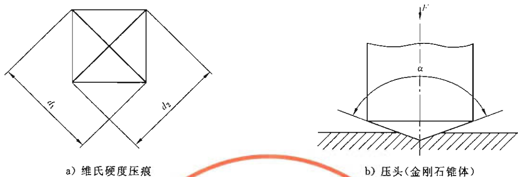
图 1 试验原理
